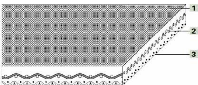
製品構造
