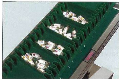
PNF-30GNとサイドウォール使用例
